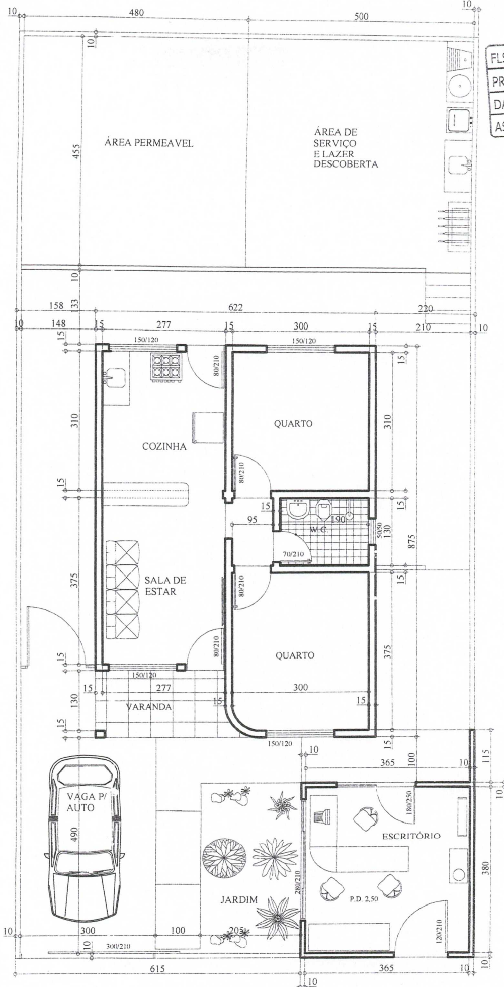
PLANTA BAIXA
